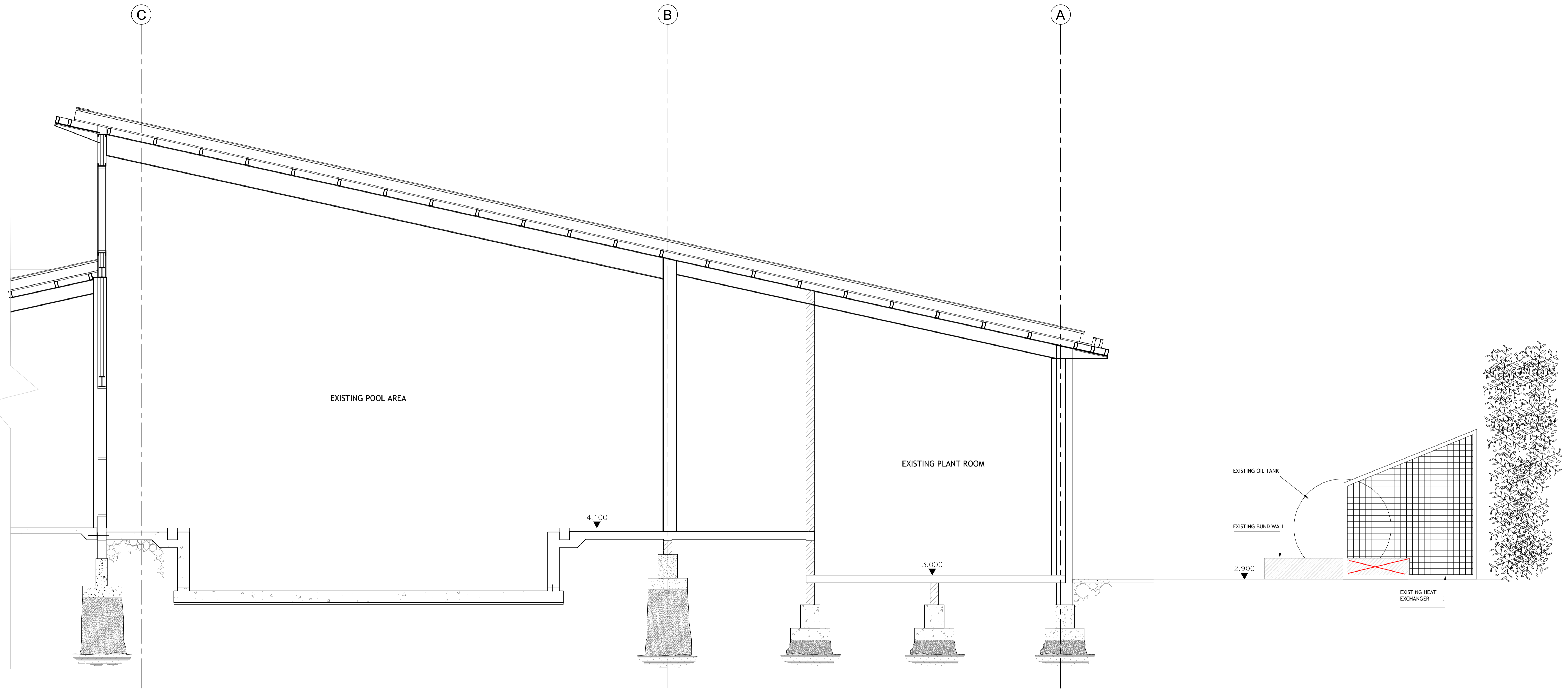
CROSS SECTION 104-01 1:50 A1 1:100 A3
