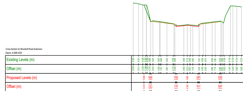
Chainage : 300.000m
