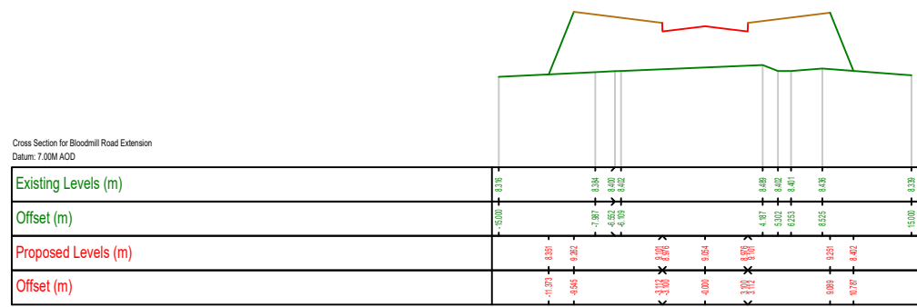
Chainage : 250.000m
