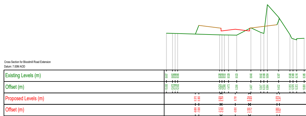
Chainage : 225.000m
