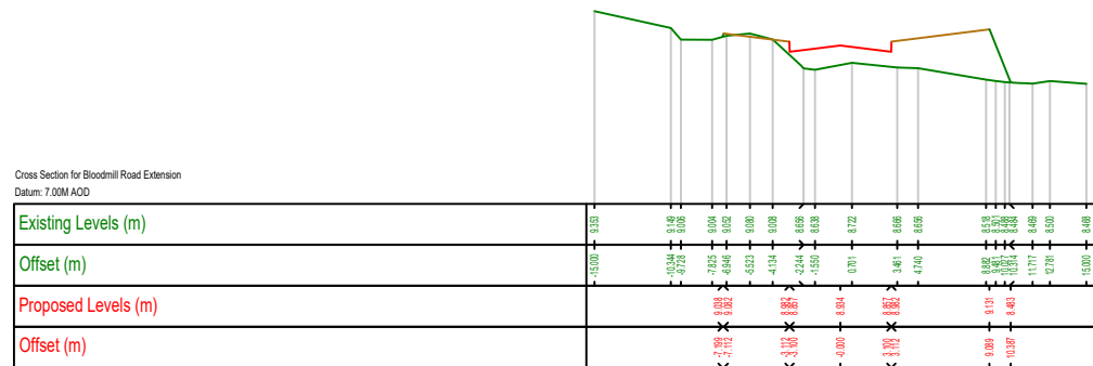
Chainage : 200.000m
