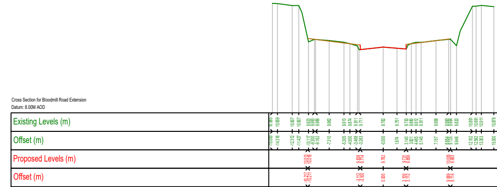
Chainage : 308.190m
